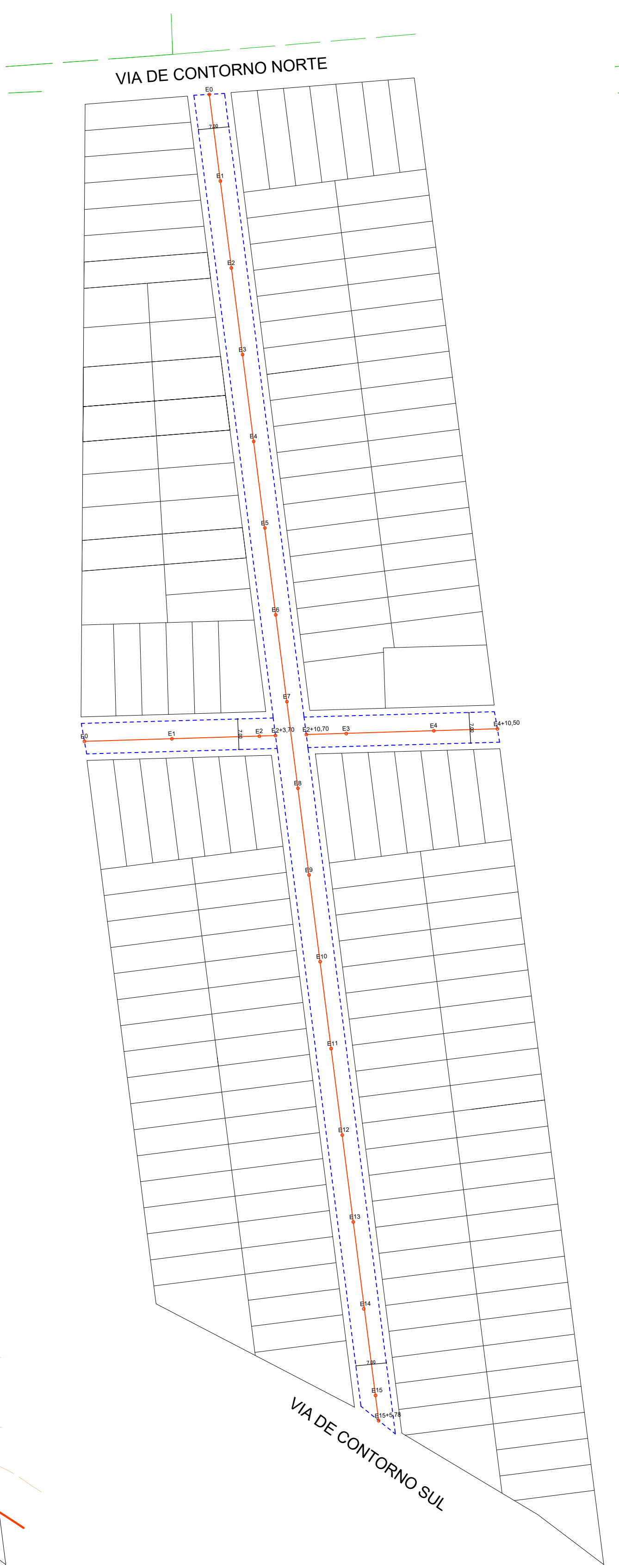
PLANTA DE ESTAQUEAMENTO ESC.: 1/500
